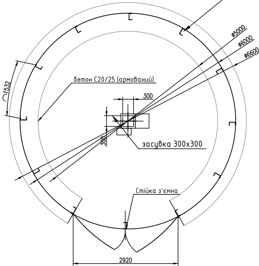
Розріз Б-Б
